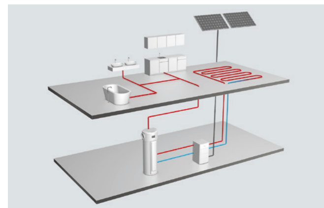
Présentation schématique du chauffage et du traitement de l'eau chaude dans une maison individuelle avec chaudière à pompe à chaleur Oertli TWH 300 et chauffage à mazout ou à gaz.
